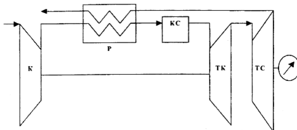
Рис. 1. Принципиальная схема двухвальной газотурбинной установки с регенерацией:
