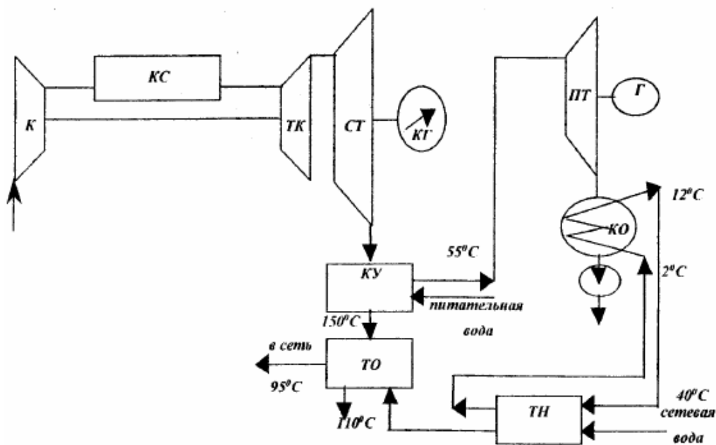
Рис. 4. Принципиальная тепловая схема установки с комбинированной утилизацией тепла уходящих газов ГТУ: К - компрессор ГТУ, ТК - турбина компрессора ГТУ, Р - регенератор ГТУ, СТ - силовая турбина ГТУ, КС - камера сгорания ГТУ, КУ - котел-утилизатор, ПТ - паровая турбина, КО - конденсатор ГТУ, ТН - теплонасосная установка, ТО - теплообменник, КГ - компрессор газа, Г - электрогенератор.
