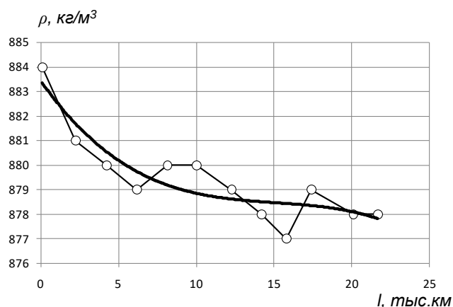
Рис. 4. Изменение плотности \rho в процессе работы моторного масла по автомобилям КАМАЗ-ЕВРО
