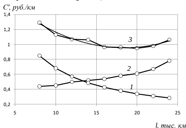
Рис. 5. Зависимость удельных затрат на замену масла (1), на текущий ремонт (2) и суммарных (3) от периодичности замены масла по автомобилям КАМАЗ-ЕВРО подконтрольной партии
