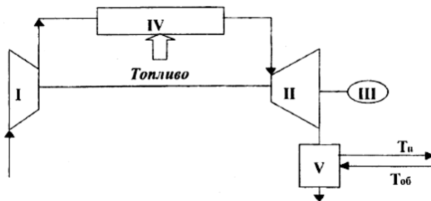
Рис. 2. Принципиальная схема газотурбинной теплофикационной установки: I - компрессор, II - турбина, III - генератор, IV - камера сгорания, V –теплообменник.
