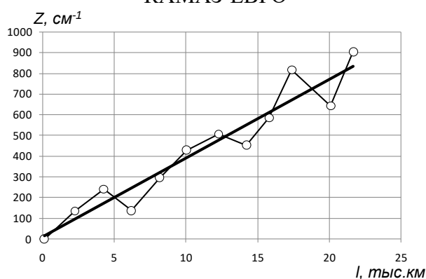
Рис. 3. Изменение загрязнённости Z в процессе работы моторного масла по автомобилям КАМАЗ-ЕВРО
