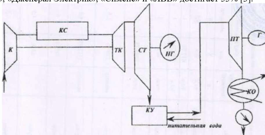
Рис.3 Принципиальная схема ПГУ с котлом-утилизатором на базе авиационного ИТД ПС-90А: К - компрессор ГТУ, ТК турбина компрессора ГТУ, СТ - силовая турбина ГТУ, КС - камера сгорания ГТУ, КУ - котел-утилизатор, ИГ - паровая турбина, КО - конденсатор ПТУ, ИГ'- нагнетатель газа, Г - электрогенератор
