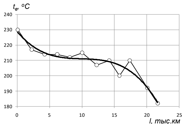
Рис. 2. Изменение температуры вспышки t_{\text{в}} в процессе работы моторного масла по автомобилям КАМАЗ-ЕВРО
