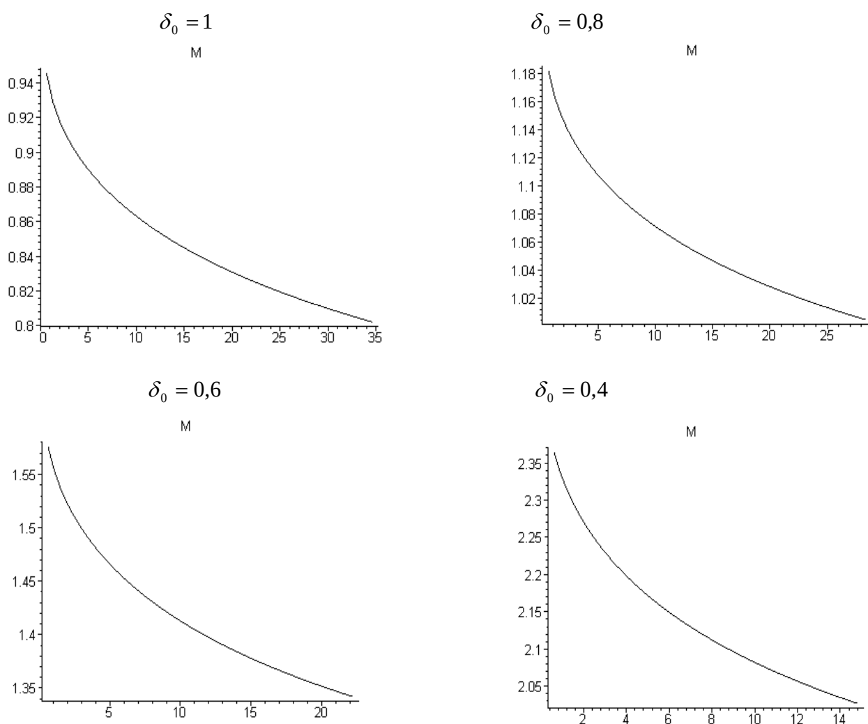
Рисунок 3. Зависимость темпа закачки раствора в пласт M (кг/с) от времени t (сек) при \delta = \mu_n / \mu_c = 0,1 различных значениях отношения \delta_0 = \mu_0 / \mu_c
