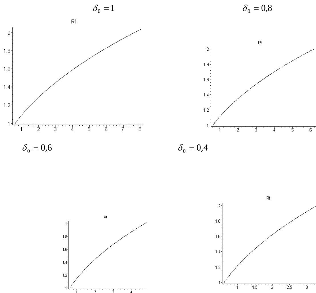
Рисунок 1. Зависимость радиуса проникания раствора в пласт R_\phi (м) от времени t (сек) при \delta = \mu_n / \mu_c = 0,5 различных значениях отношения \delta_0 = \mu_0 / \mu_c
