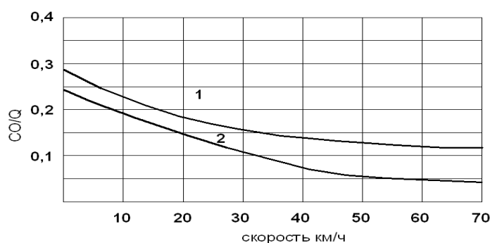
Рисунок 2 – График зависимости \gamma_{CO} от скорости потока V
