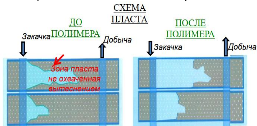
Рисунок 1 – Теоретическая схема пласта до и после полимерного заводнения
