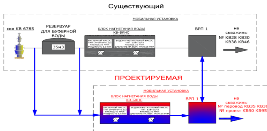
Рисунок 1 – Проектная схема расширения существующей системы водонагнетания на месторождении Карабулак
