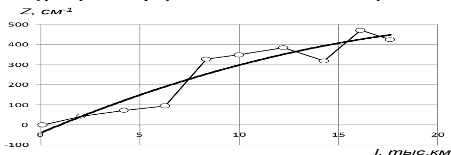
Рис.1. Изменение загрязненности Z в процессе работы моторного масла по автомобилям КАМАЗ 4311.
