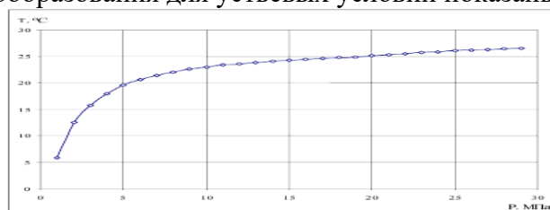
Рисунок 1 – Равновесные параметры гидратообразования газа со скважин Тенгизского месторождения
