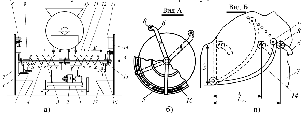
а) схема кормораздатчика; б) вид А; в) вид Б:
