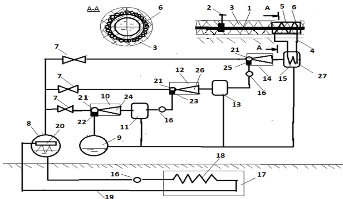
Сурет. 1. Көліктік жылытылатын құбырдың сызбасы:
