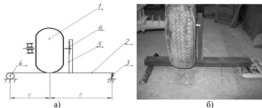
а) схема установки; б) общий вид; 1 – пневматическая шина; 2 – рычаг; 3 – весовое устройство; 4 – шарнир; 5 – линейка; 6 – указатель высоты
