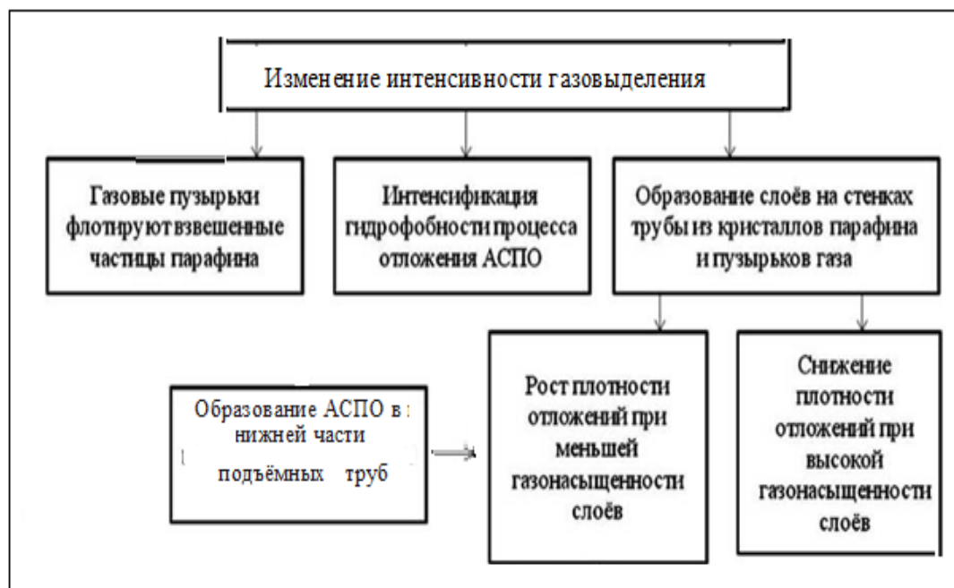
Рисунок 3. Выявление характера влияния газовыделения на процесс образования АСПО.
