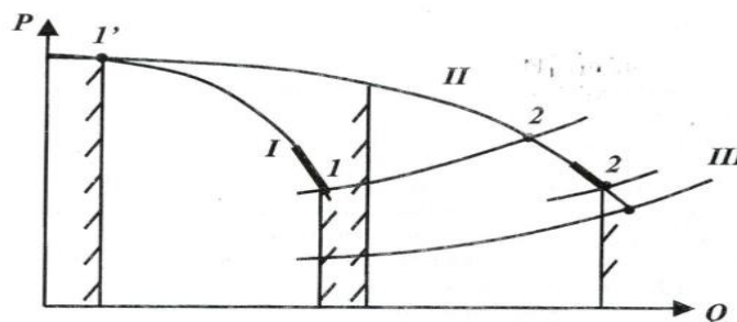
Рисунок 2 – Согласование характеристик сети и КНС при ТДЗ
