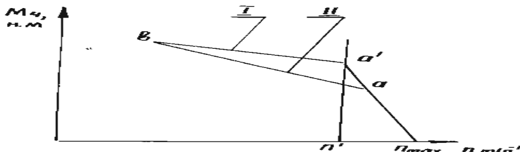
1-сурет Қозғалтқыштың жылдамдық мінездемесі
