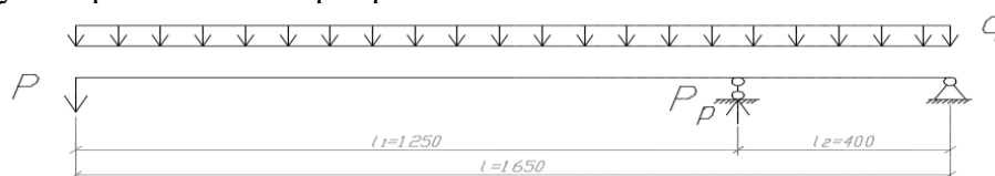
Рисунок 3 – Расчетная схема определения разрушающей нагрузки
