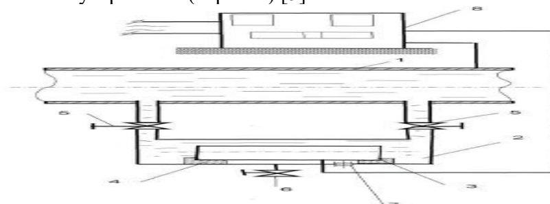
Рисунок 1 – Схема устройства для защиты трубопровода от гидратоотложений : 1 – трубопровод; 2 – байпас; 3 – расходуемый анод; 4 – упор; 5 – задвижки комммутирующие; 6 – вентиль дренажный; 7 – устройство уплотнения; 8 – станция катодной защиты
