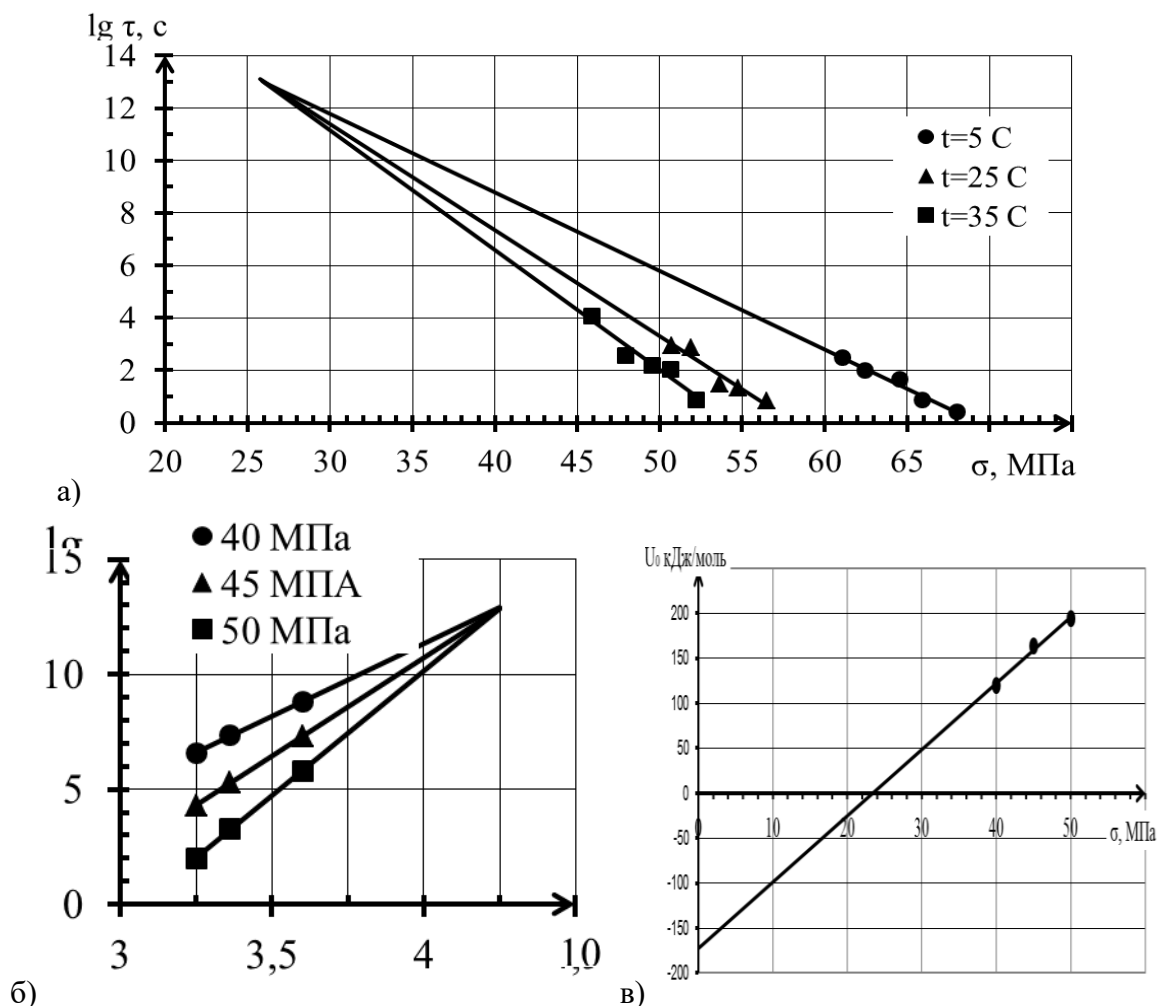
а – зависимость логарифма долговечности от напряжения; б – зависимость логарифма долговечности от обратной температуры увеличенной в 1000 раз; в – зависимость энергии активации процесса разрушения от напряжения
