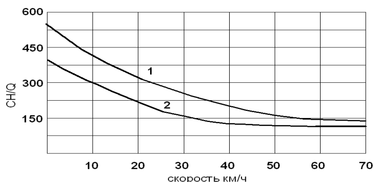
Рисунок 3 – График зависимости \gamma_{CH} от скорости потока V
