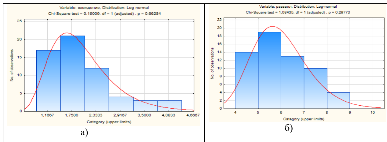
Рисунок 3 – Гистограммы и теоретические кривые законов распределения: а) – схождения колес; б) – развала колес.
