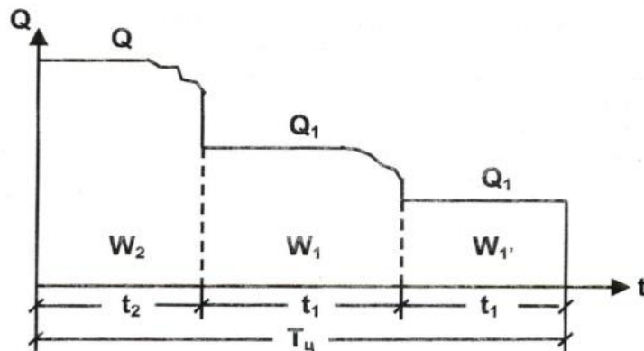
Рисунок 2 – Согласование характеристик сети и КНС при ТДЗ
