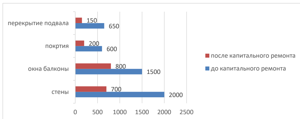
Рисунок 3. Удельные тепловые потери через ограждающие конструкции, Вт/К
