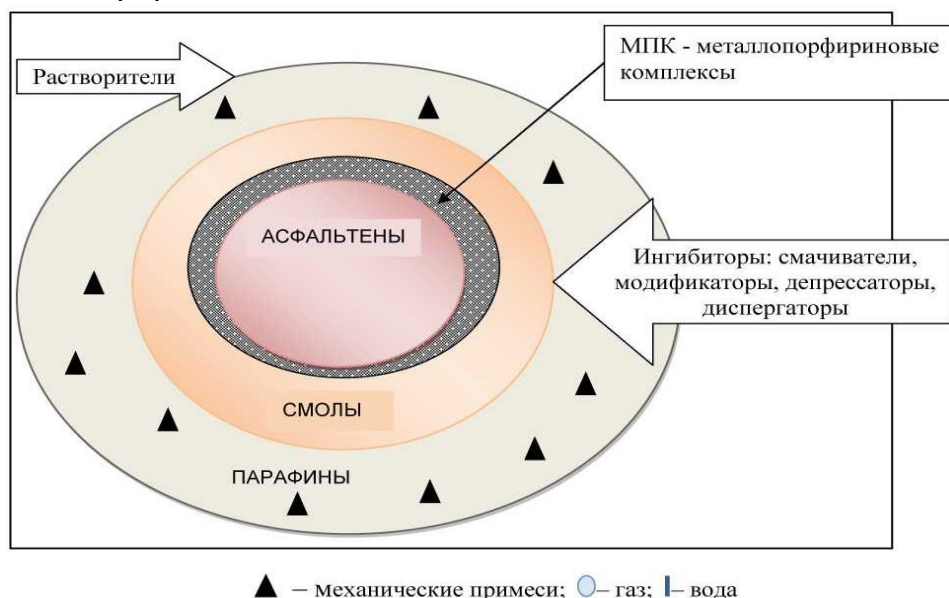
Рисунок 1. Конфигурация агломерата АСПО.
