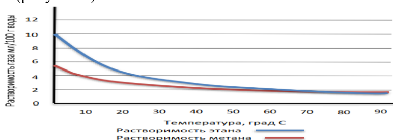
Рисунок 1 – Растворимость некоторых газов в воде при нормальных условиях
