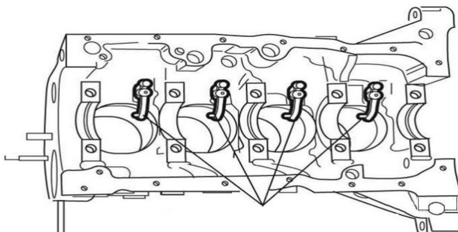
Рис.2. Установка маслофорсунки в масляную магистраль
