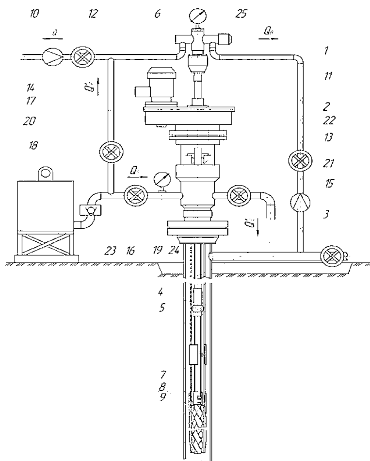
Сурет 1. Күрделі жағдайларда мұнай өндіру үшін штангалық бұрандалы сорғыны орнату.
