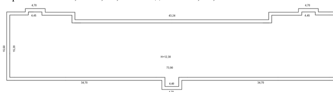
Рисунок 1. Наружные обмеры здания
