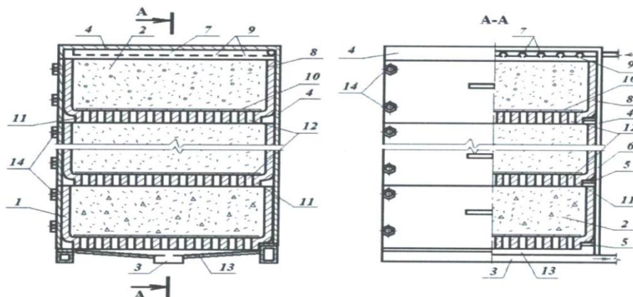
1-сурет. Жылжымалы кассеталары бар көп құрамды сорбциялық сүзгі:
